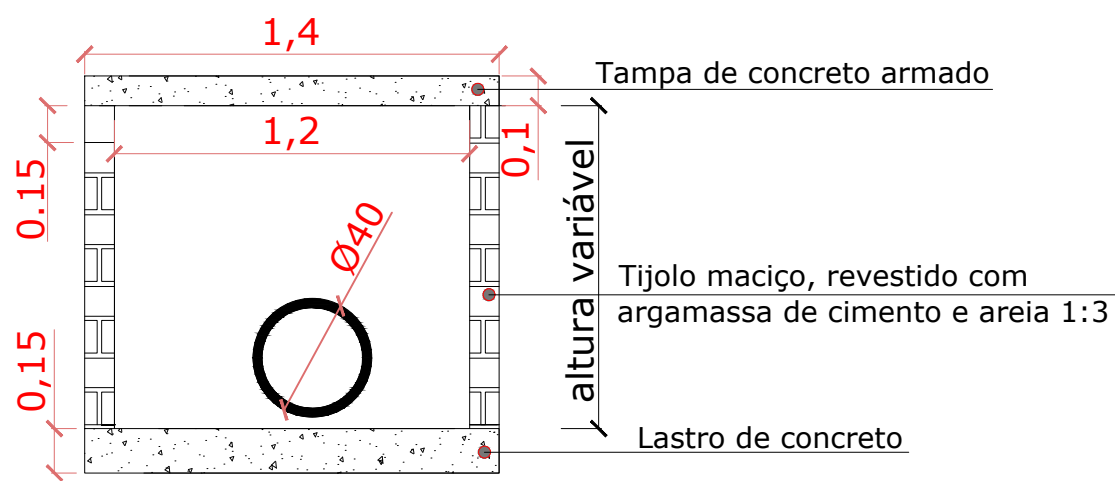
CAIXA TIPO BOCA DE LOBO ESC. 1/25
